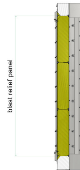
A-A section
